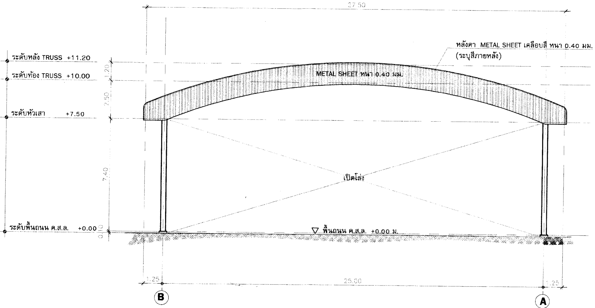
รูปด้าน 3 มาตรฐาน 1:100
