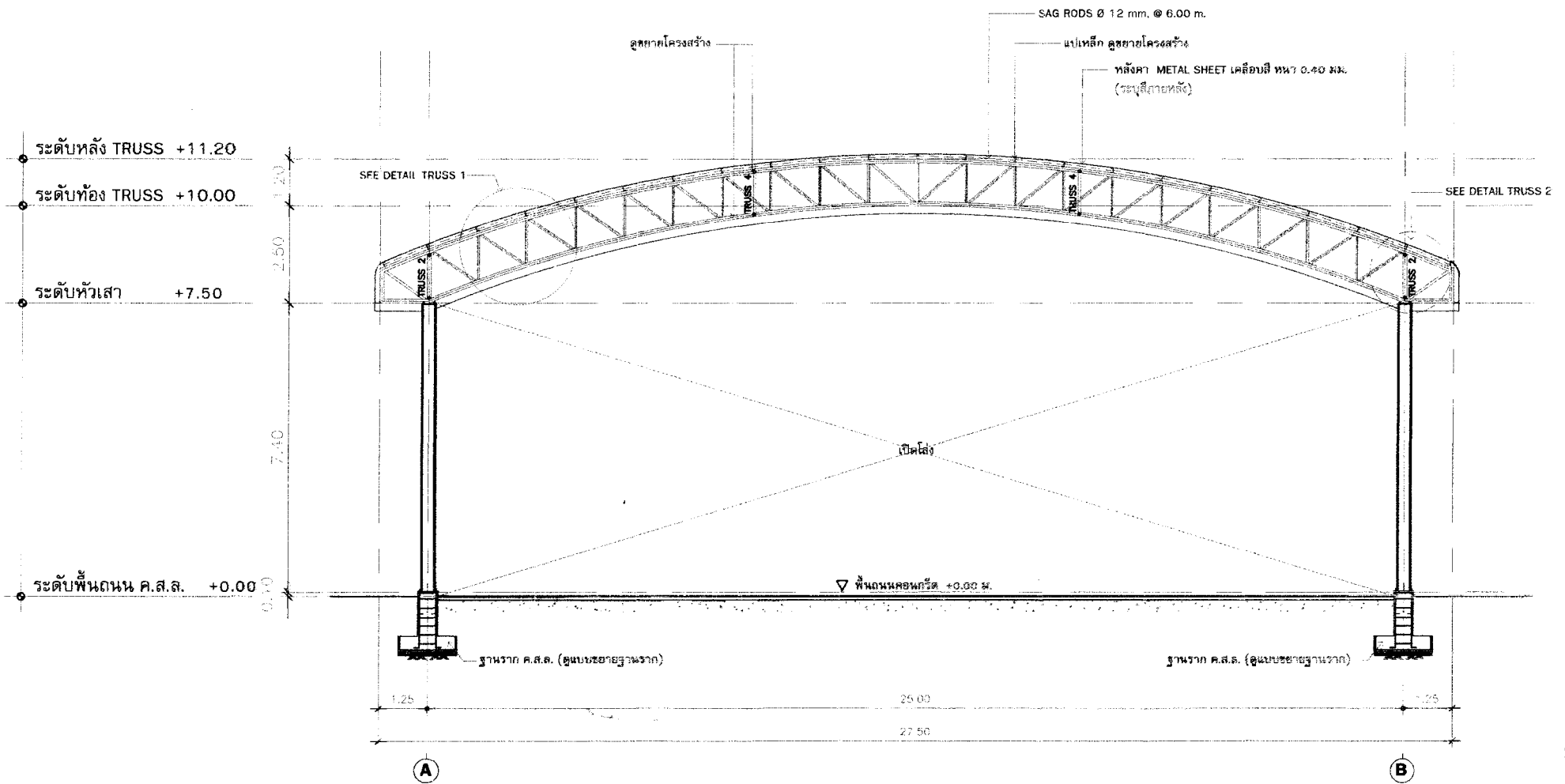
รูปตัด A มาตรฐาน 1:100
