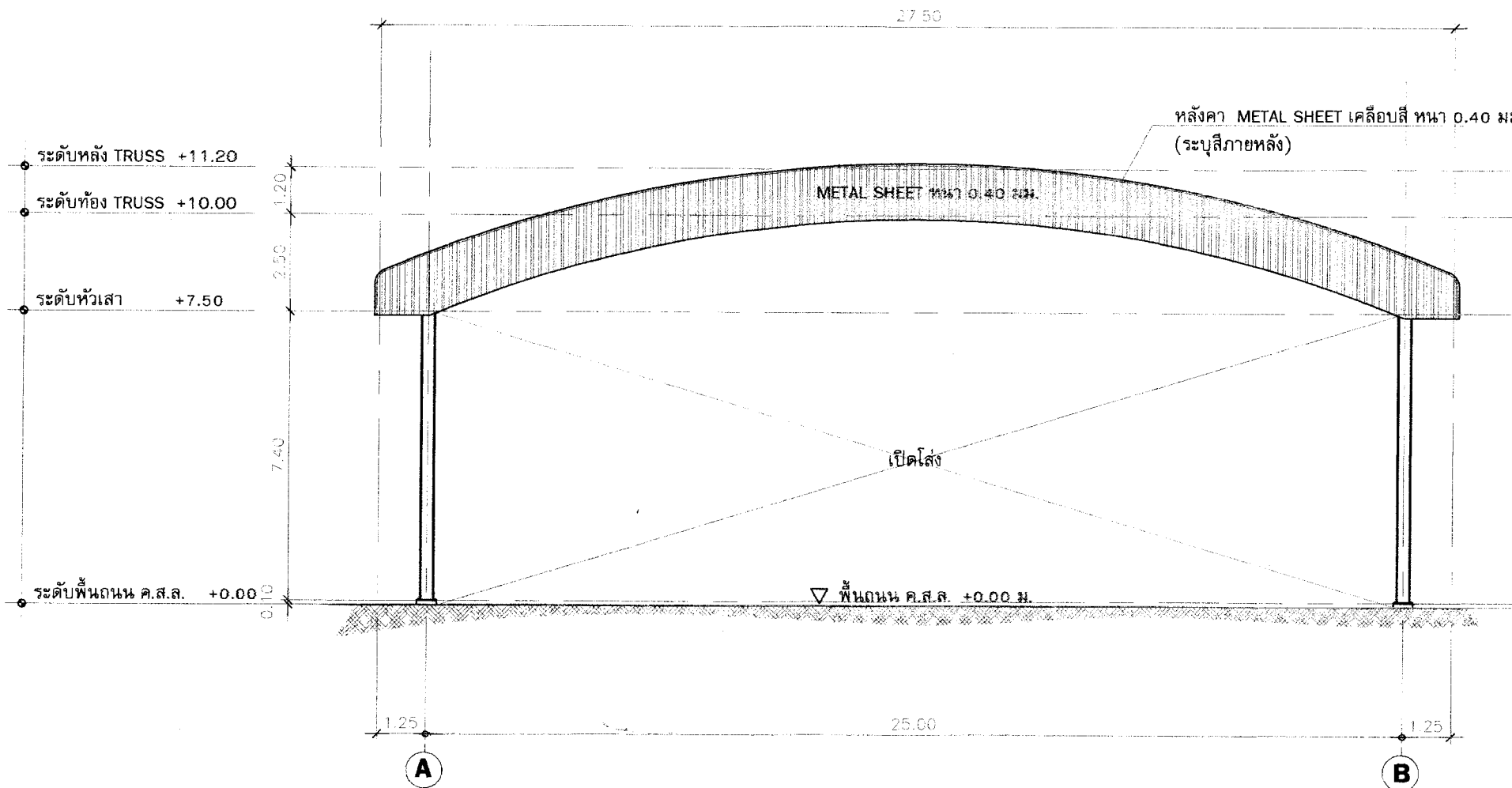
รูปด้าน 1 1 1:100
