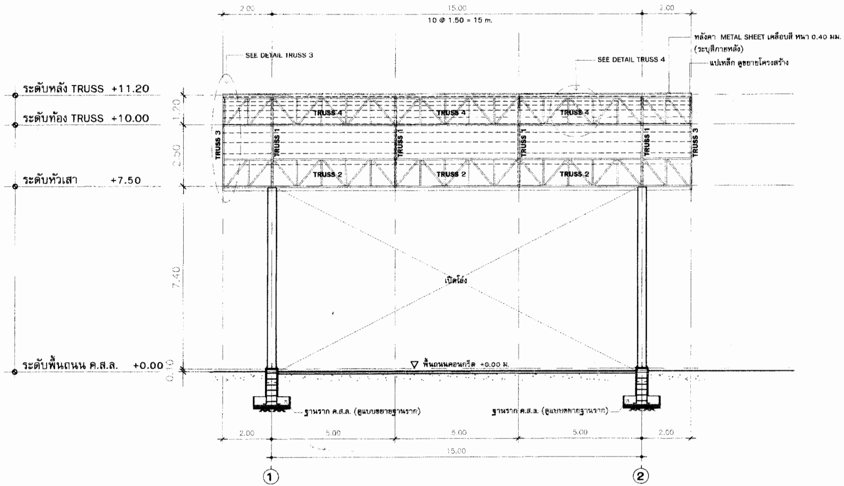
รูปตัด B มาตรฐาน 1:100
